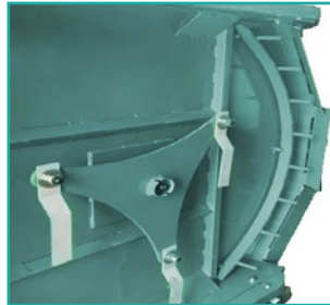
Brana za zadržavanje biljnih ostataka radi boljeg usitnjavanja The barrage for retention of crop residue for better fragmentation
