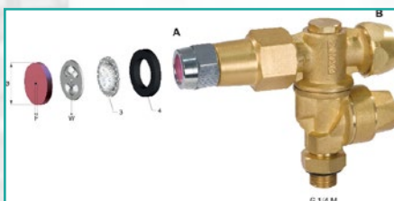
Top dizna Top nozzle
