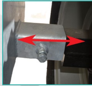
Osovina podesiva po širini Width adjustable axle
