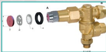
Top dizna Top nozzle
