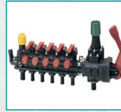
Proporcionalni distributor sa 5 jedinica Proportional distributor with 5 ways
