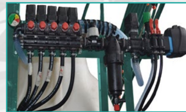
Elektronska komandna grupa Electronic control unit
